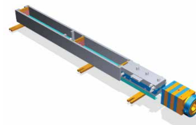
Khuôn đùn nhựa Plastic extrusion mold
