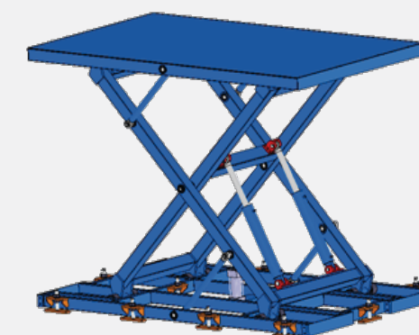
Bàn nâng hạ Lifting table
