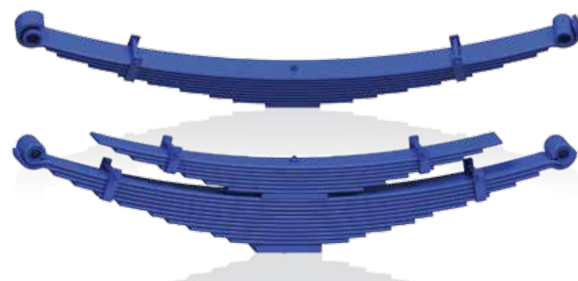
Nhíp xe tải tải trọng 7,000 - 7,250 kg Leaf springs of truck 7,000 - 7,250 kgs
