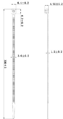
Cable Tie 3.6*300mm Color: Custom
