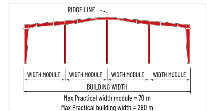
Multi-Span "3" (MS-3)
