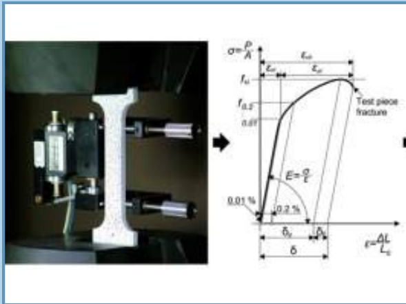
Tensile Test
